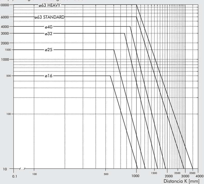
Carga L (N) Diagrama de carga admisible
